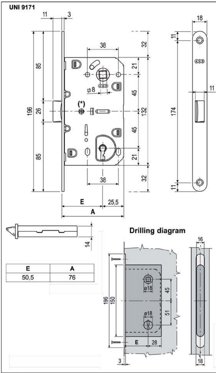
Γ1. Κλειδαριά πόρτας εσωτερικού χώρου AGB Medianna evolution 18
