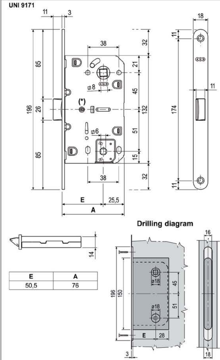
Γ2. Κλειδαριά πόρτας λουτρού (WC) AGB Medianna evolution 18
