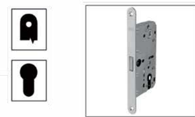
Ασφαλείας Δ2. Μαγνητική ασφαλείας AGB Polaris 18
